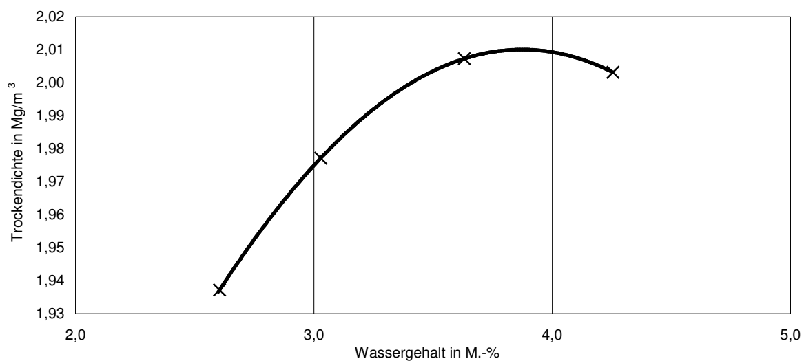
Proctorkurve des Baustoffgemisches 0/32 (STS) gemäß Prüfzeugnis Nr. 45797SoB/24 vom 31.01.2025
