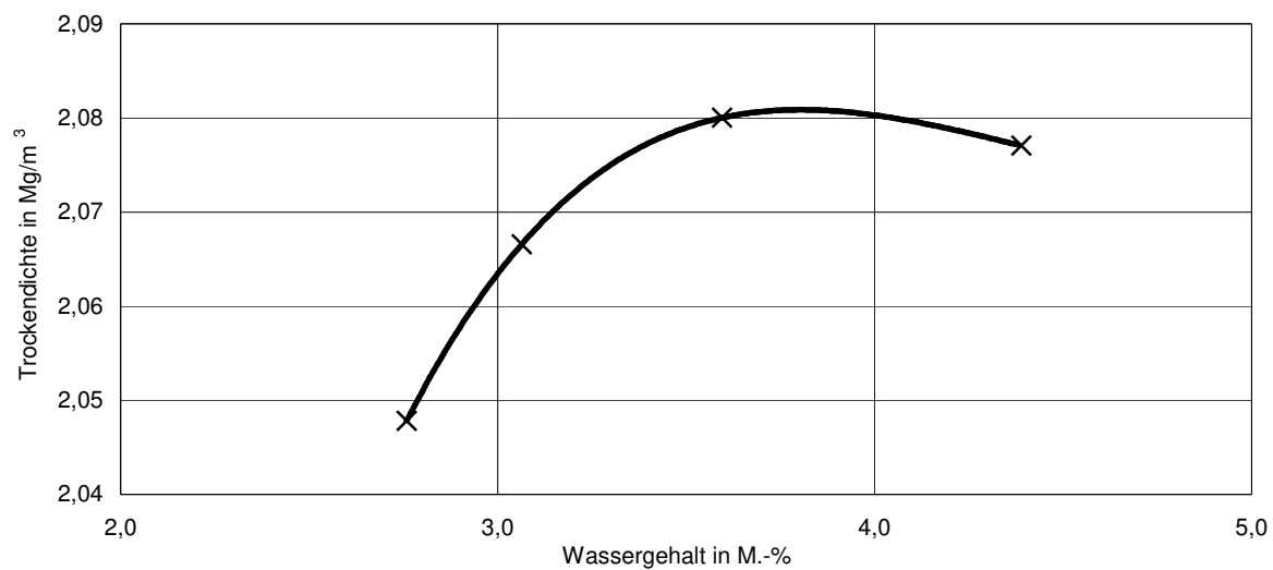
Proctorkurve des Baustoffgemisches 0/45 (FSS - UF 3) gemäß Prüfzeugnis Nr. 45801SoB/24 vom 31.01.2025
