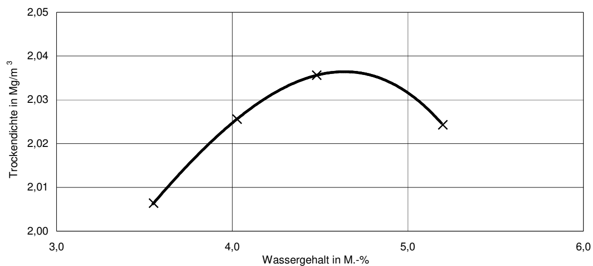
Proctorkurve des Baustoffgemisches 0/32 (FSS) gemäß Prüfzeugnis Nr. 45798SoB/24 vom 31.01.2025
