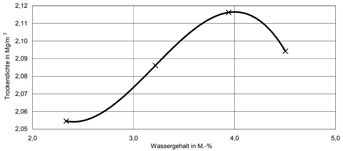
Proctorkurve des Baustoffgemisches 0/45 (STS) gemäß Prüfzeugnis Nr. 42784SoB/21 vom 17.01.2022
