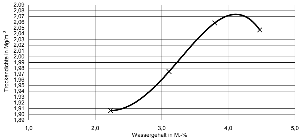
Proctorkurve des Baustoffgemisches 0/45 (STS) gemäß Prüfzeugnis Nr. 40175SoB/19 vom 25.06.2019
