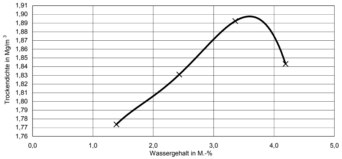
Proctorkurve des Baustoffgemisches 0/32 (FSS) gemäß Prüfzeugnis Nr. 40174SoB/19 vom 25.06.2019
