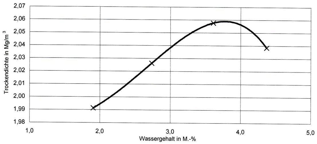
Proctorkurve des Baustoffgemisches 0/45 (STS) gemäß Prüfzeugnis Nr. 39231SoB/18 vom 25.06.2018
