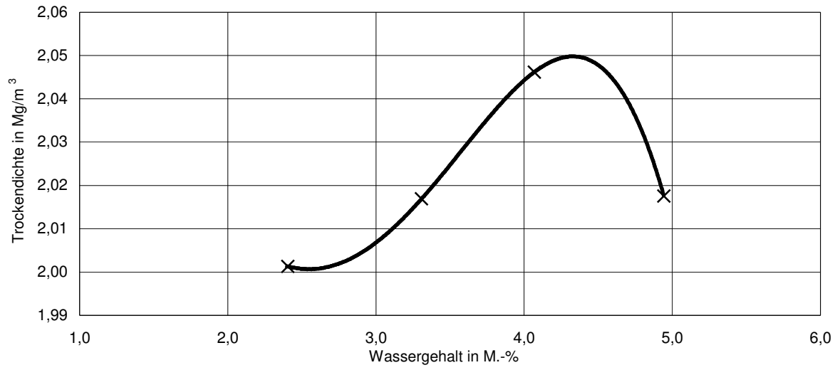
Proctorkurve des Baustoffgemisches 0/45 (STS) gemäß Prüfzeugnis Nr. 43817SoB/22 vom 23.02.2023
