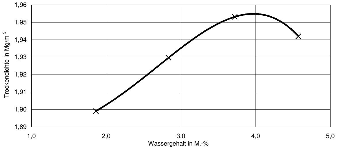
Proctorkurve des Baustoffgemisches 0/32 (FSS) gemäß Prüfzeugnis Nr. 43816SoB/22 vom 23.02.2023
